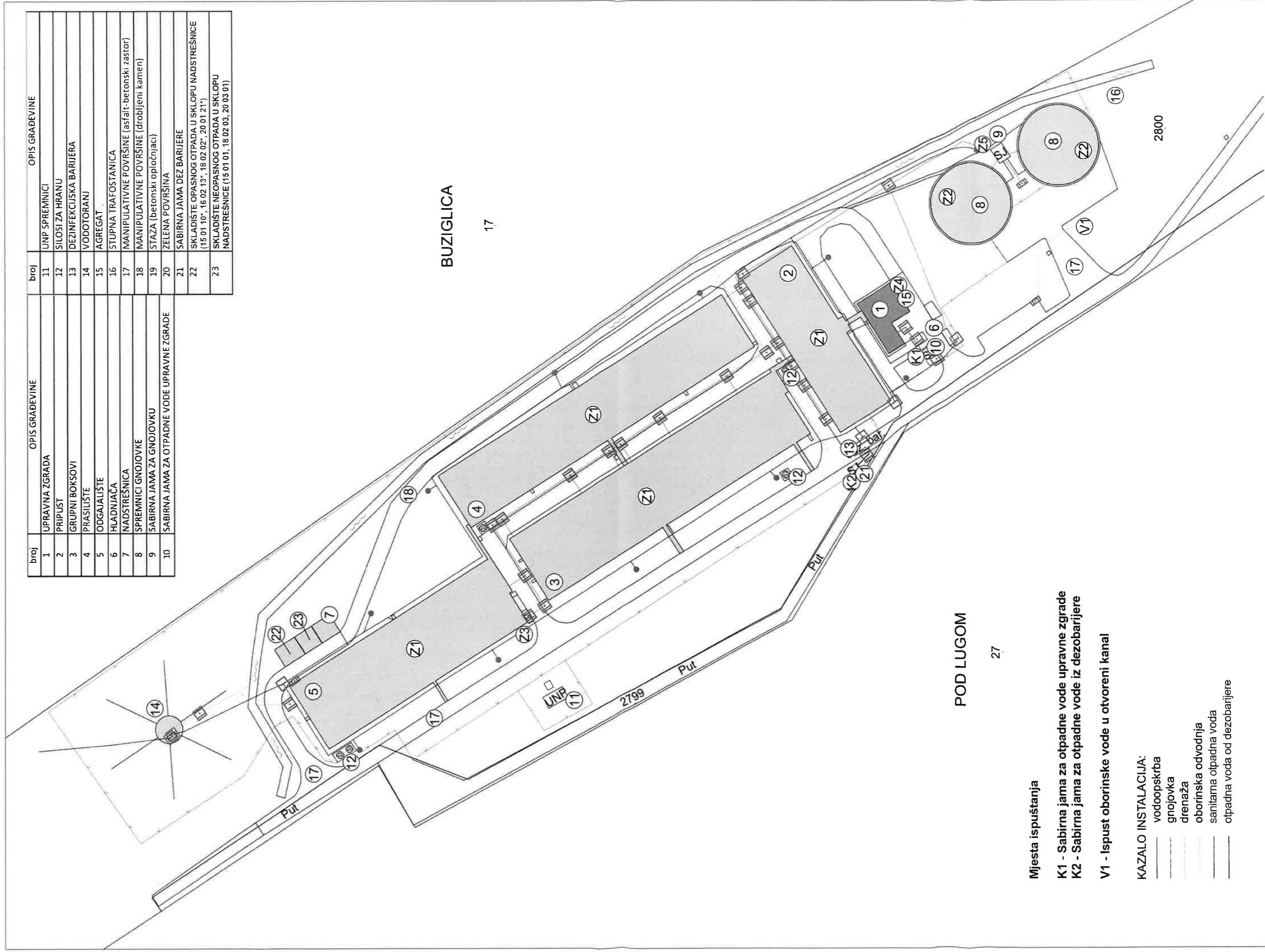
Prilog 1. Situacija s prikazom objekata, mjesta emisija i sustava vodoopskrbe te odvodnje otpadnih voda na lokaciji farme Podlugovi
